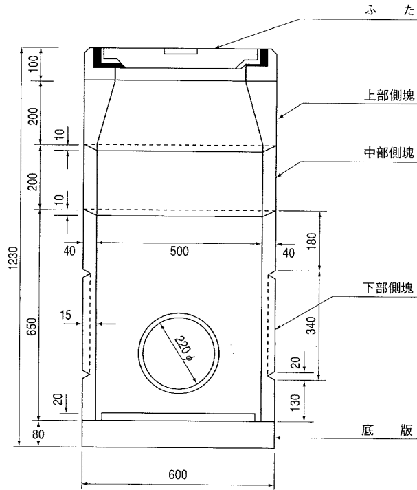
組立図 (φ500用)
