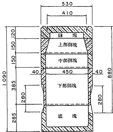
組立図
