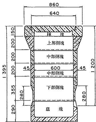
組立図
