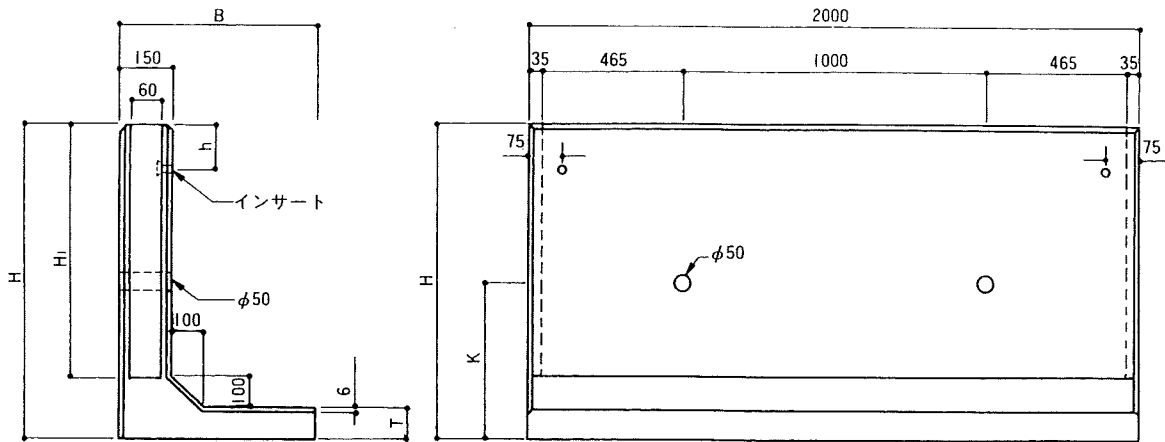
寸法表
