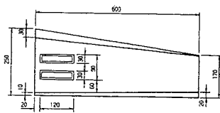
歩車道平 (A, B 共通)
