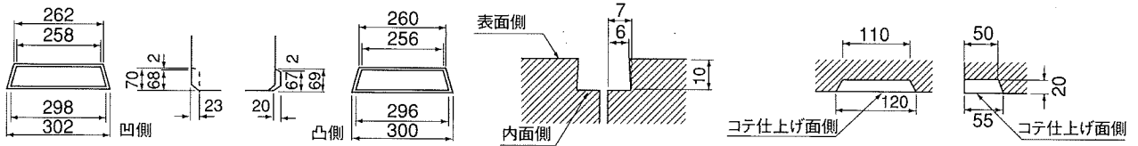
接合部詳細図
