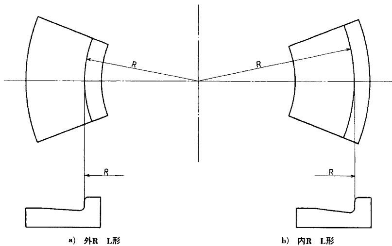
附属書5参考図1 曲率半径の取り方
