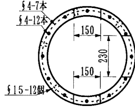
浸透側塊 (有孔)
