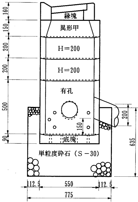
雨水浸透柵構造図
