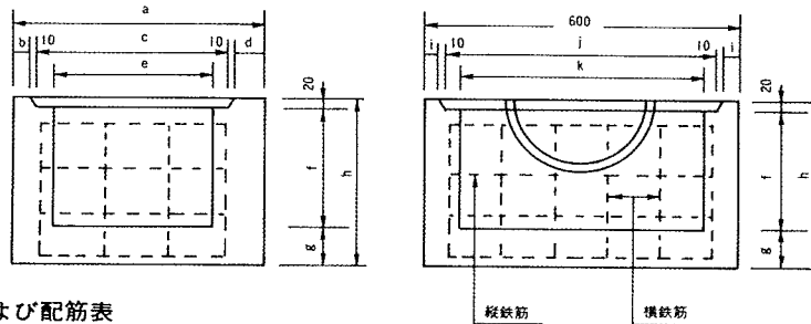
上部側塊寸法および配筋表
