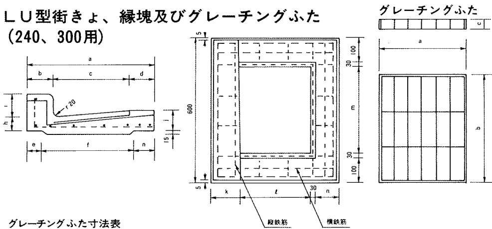
グレーチングふた寸法表
