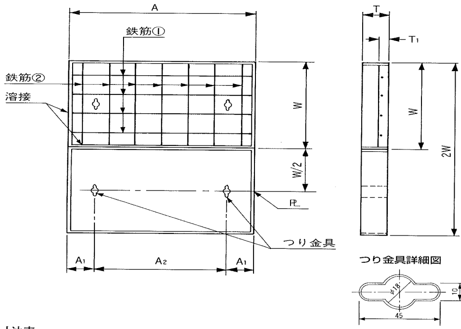
寸法表
