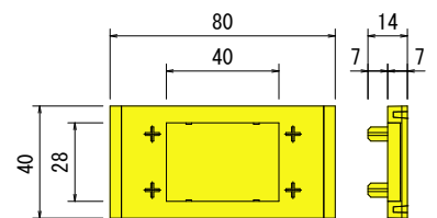
反射板詳細図
